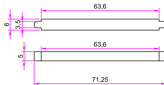
SPACER
